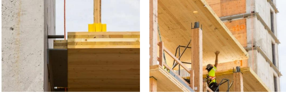
Şekil 14: Betonarme-ahşap hibrit sistem uygulaması örneği. (Law, 2016)
