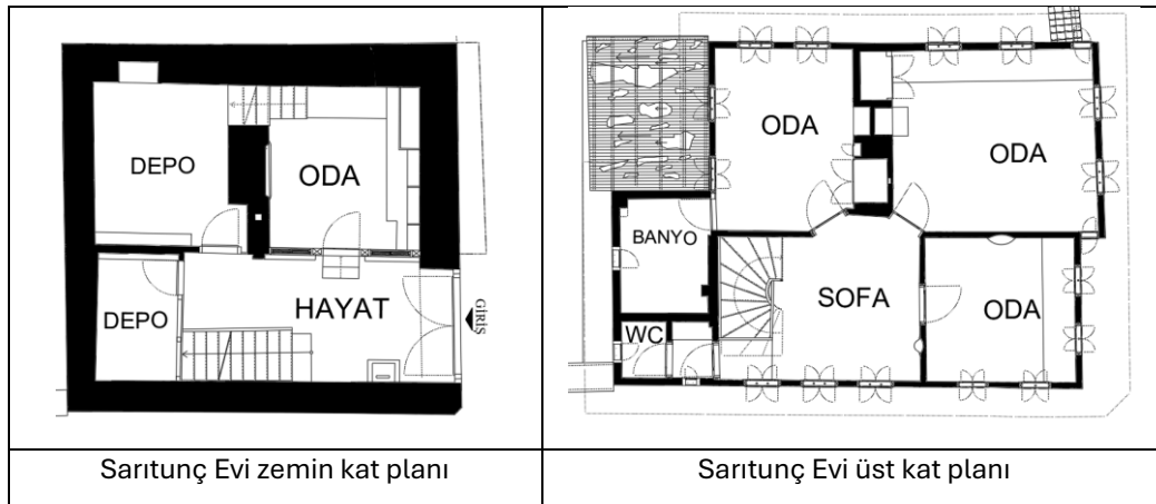
Şekil 5. Sarıtunç Evi'ne ait kat planları (Mimar Elif Hacıoğlu'ndan düzenlenmiştir)
