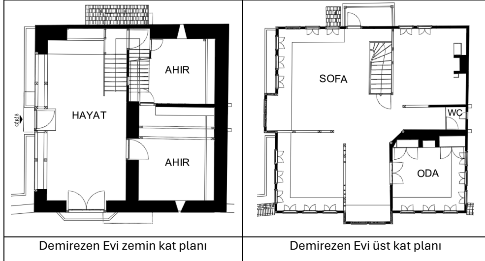
Şekil 4. Demirezen Evi'ne ait kat planları (Mimar Elif Hacıoğlu'ndan düzenlenmiştir)
